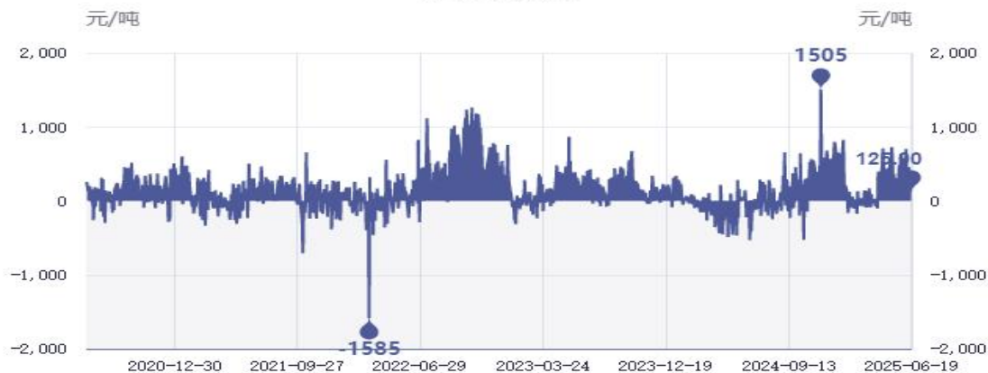
锌基差走势
